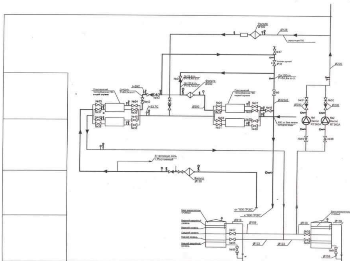
Рис. 3.2. Технологическая схема ПНС (контур ГВС)
