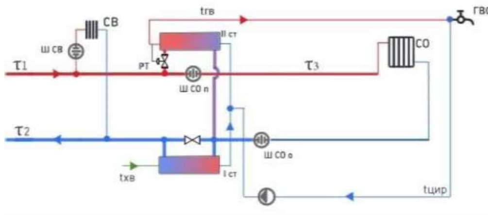
Рис. 2. Двухступенчатая (смещенная) схема присоединения подогревателей ГВС с зависимым присоединением системы отопления
